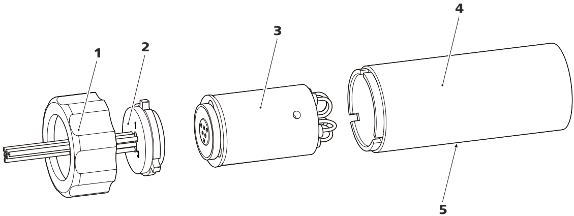
图 23 Metrohm Suppressor Module (万通抑制模块 MSM) 的部件
