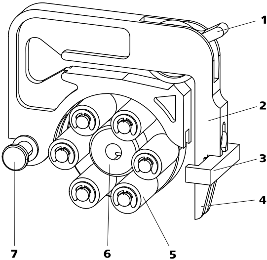
图 14 蠕动泵
